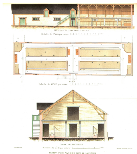
Élévation, plan et coupes longitudinale et transversale d'une vacherie pour 40 laitières
